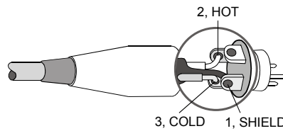
Abbildung 2.1: Symmetrische Beschaltung des Eingangs
